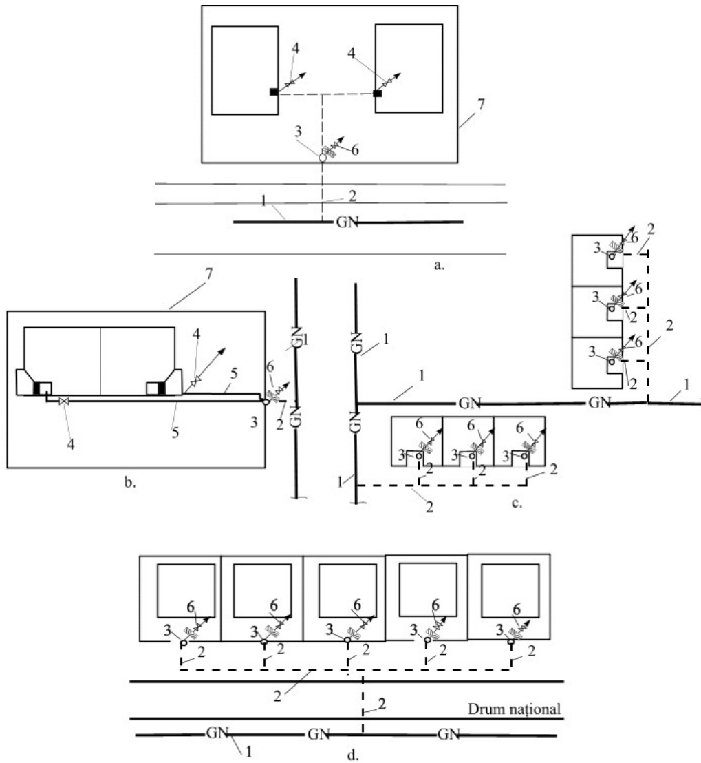
Fig. 11 Schemă de principiu privind alimentarea prin branșament comun și ramificat
